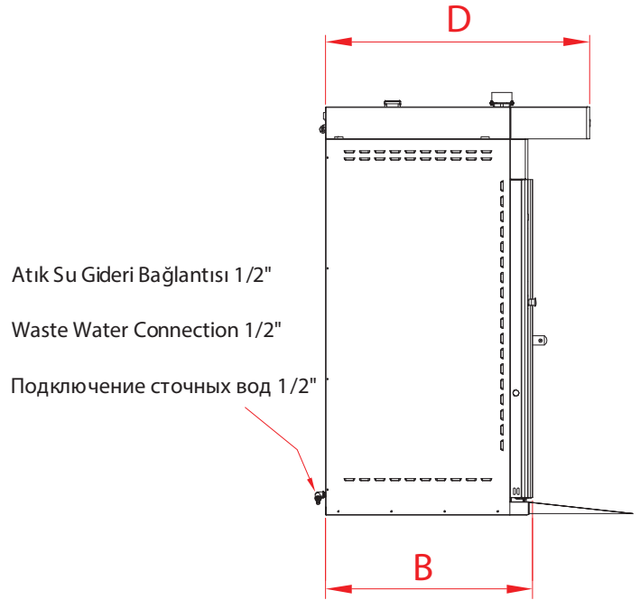
Sol Yan Görünüş - Left Side View - слева Вид сбоку
